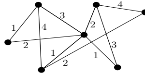
Figura 2.9: Coloración de Grundy para una gráfica con |V(G)| = 7 .
