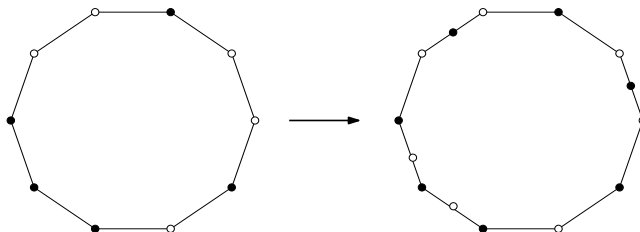
Figura 3.7: Gráfica alternante generada de G arbitraria.
