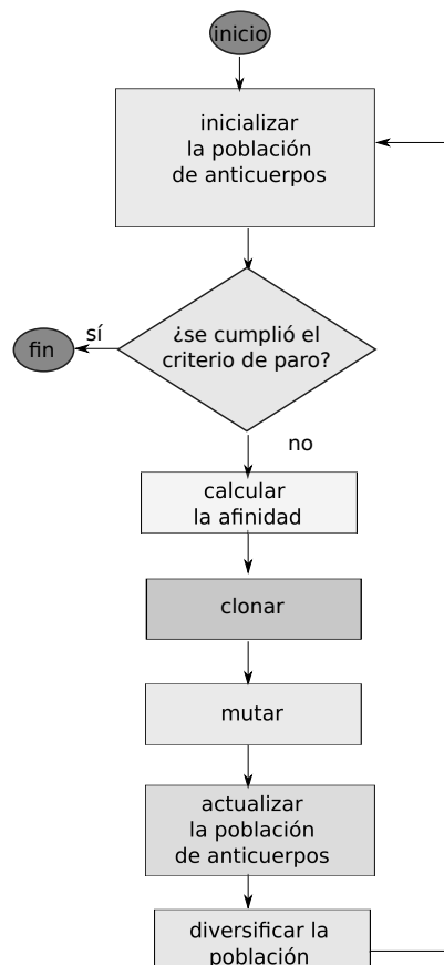
Figura 2.11: Algoritmo general de selección clonal
