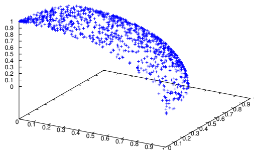
Figura A.8: Frente de Pareto verdadero de DTLZ3
