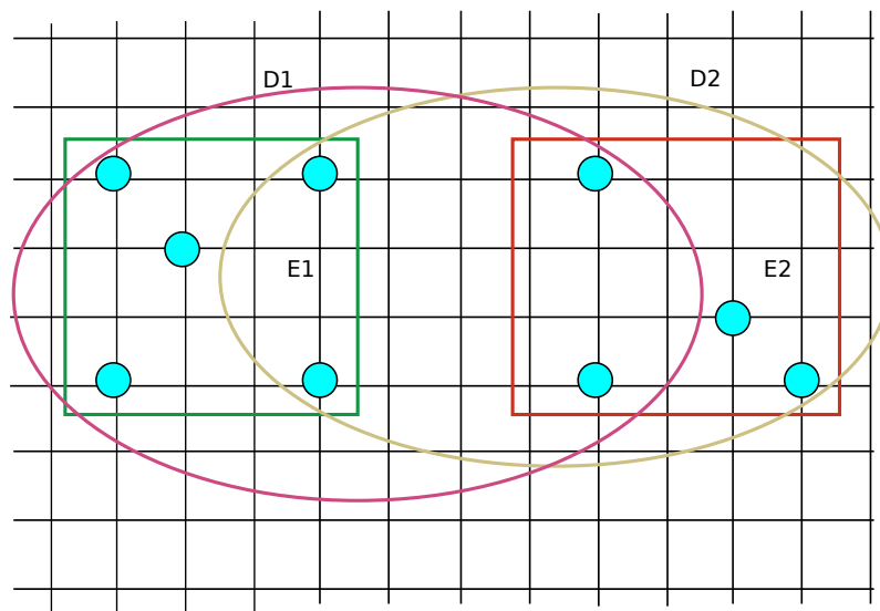
Figura 4.3: Cúmulos estrictos vs difusos
